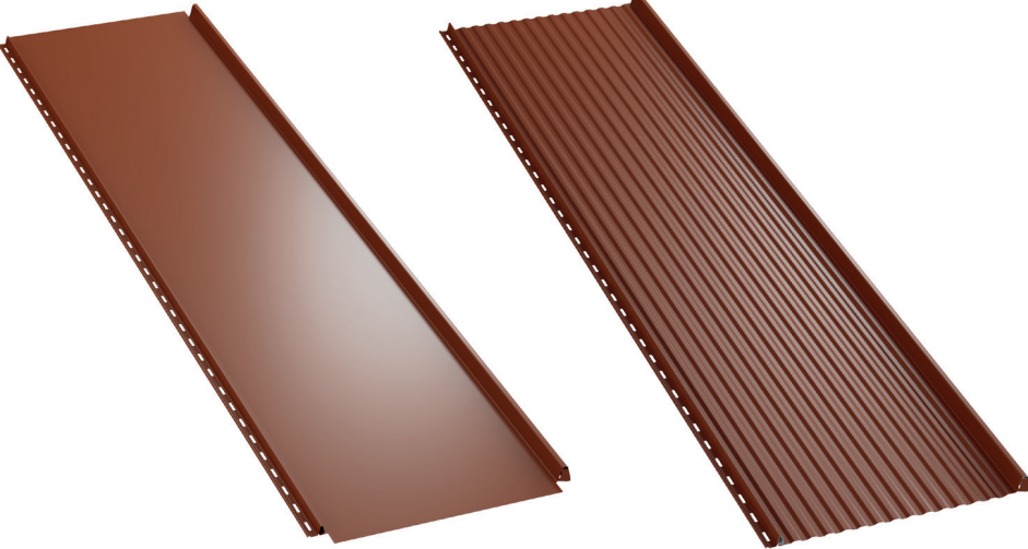
plaski profilowany Szerokość całkowita 511 mm Szerokość całkowita 500 mm Szerokość krycia 477 mm Szerokość krycia 466 mm
