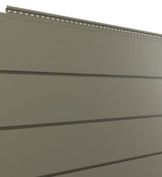
P05 » z prostą fugą, naroże kątowe Szerokość całkowita 306 mm Szerokość krycia 260 mm
