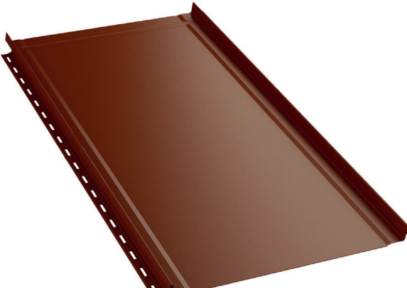
Savoy » Szerokość całkowita 524 mm Szerokość krycia 484 mm
