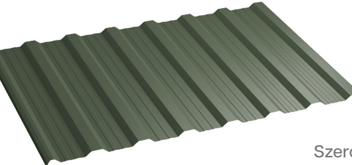
T-18 » Dach Szerokość Szerokość Elewacja całkowita krycia 1 160 mm 1 120 mm 1 166 mm 1 120 mm
