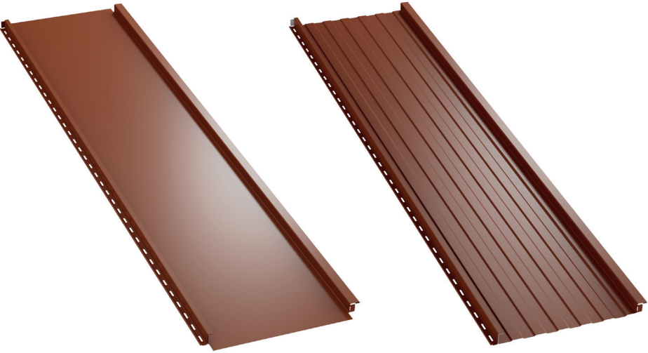
plaski profilowany Szerokość całkowita 484 mm Szerokość całkowita 479 mm Szerokość krycia 446 mm Szerokość krycia 441 mm
