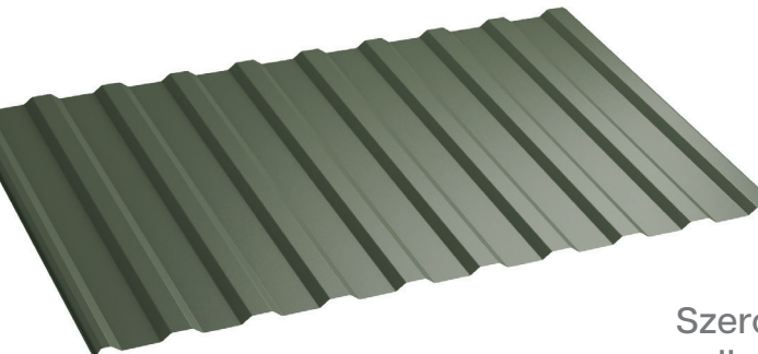
T-14 » Dach Szerokość Szerokość Elewacja całkowita krycia 1 169 mm 1 130 mm 1 174 mm 1 130 mm
